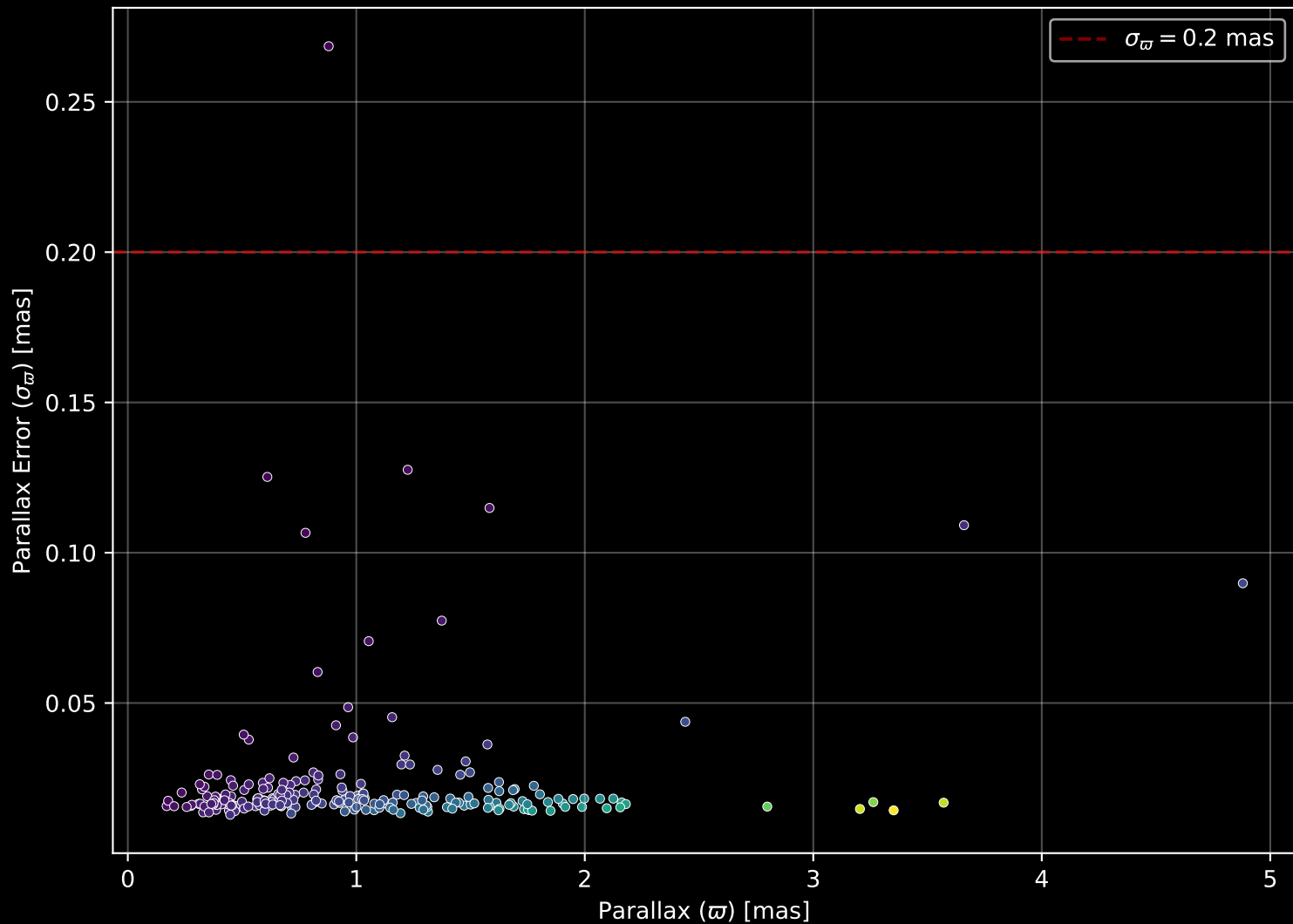
GALAH DR4 Field: [9272] Parallax Quality (n= 231)
