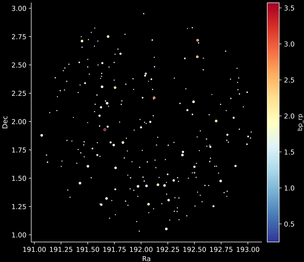
GALAH DR4 Field: [9272] Stars: 231
