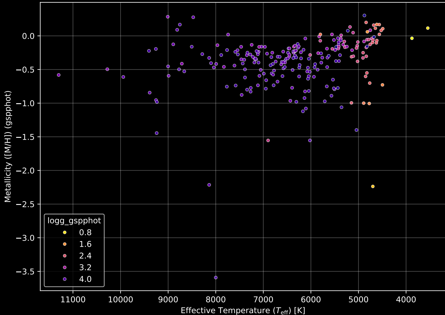
GALAH DR4 Field: [9272] Stellar Population Parameters (n= 231)
