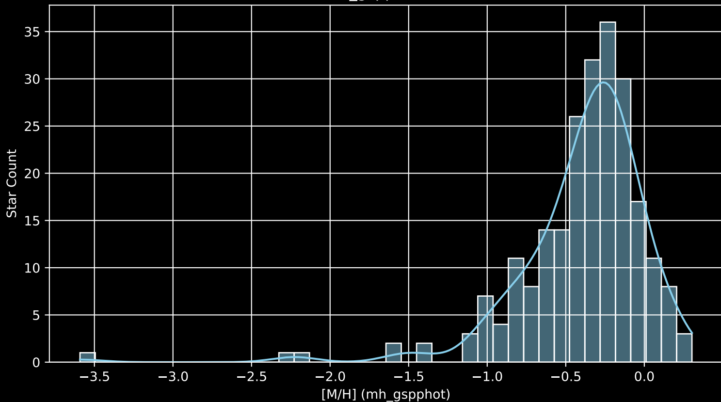
GALAH DR4 Field: [9272] [M/H] (mh_gspphot) (n= 231)
